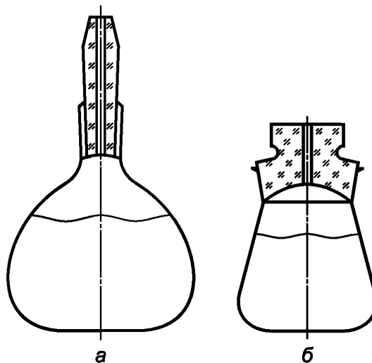
Рисунок 2 — Стекланный пикнометр
