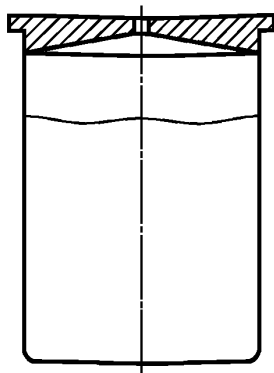
Рисунок 1 — Металлический пикнометр
